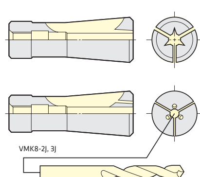
Schneidwerkzeug ohne Innenkühlung
