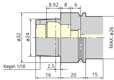
HSK32E (DIN69893-5)
